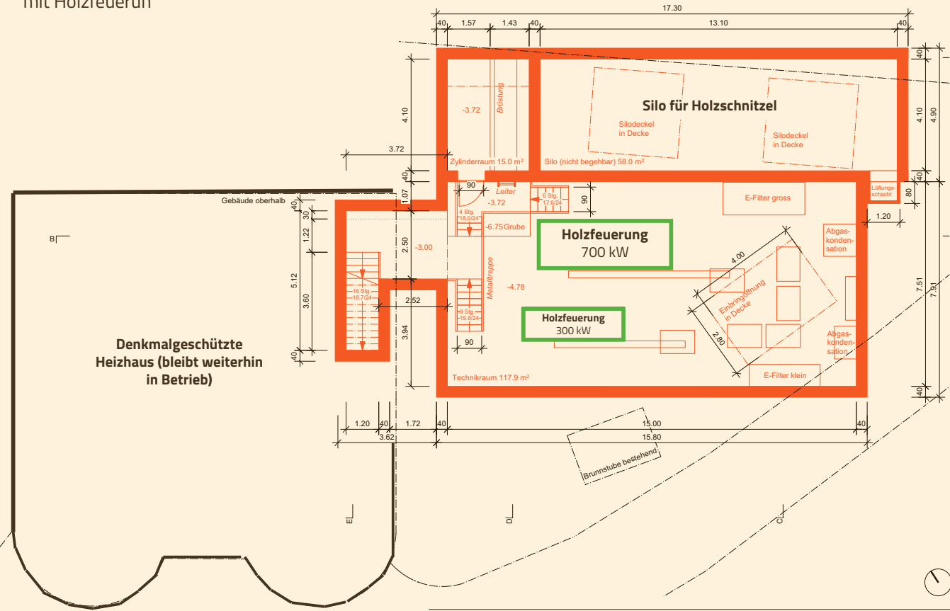
Bild 5: Bauplan - Heizhaus mit Holzfeuerun
